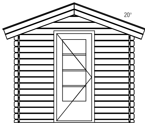
Voor aanzicht / Front view / Vorderansicht
